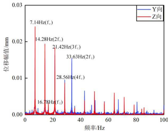
图 9 保持架质心径向位移频谱
