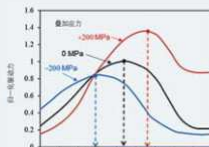
受叠加应力影响的球型夹杂物引发的裂纹扩展驱动力
