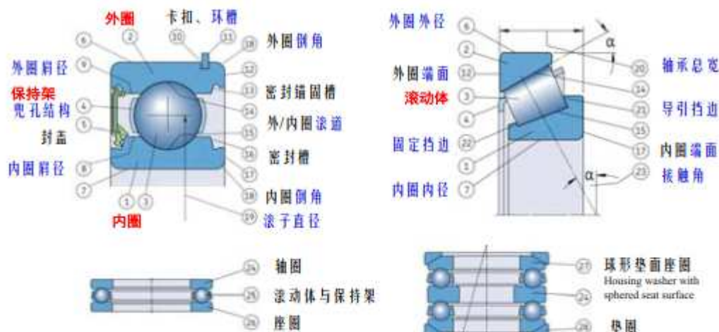
主要设计对象与设计参量
